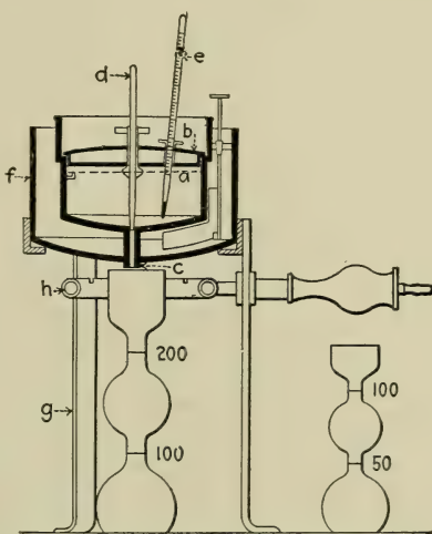
FIG. 158.—Engler Viscosimeter.
